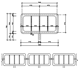
Typy zábran.
